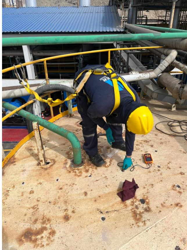
FIG. N°8: Trazado de cuadrículas para los puntos de medición en techo de tanque.
