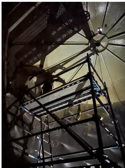
FIG. N°10: Medición de espesor en estructura de tanque de almacenamiento.
