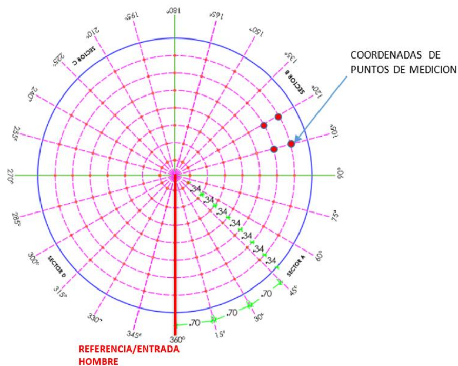
FIG. N°7: Distribución de puntos de medición en techo de Tanque.
