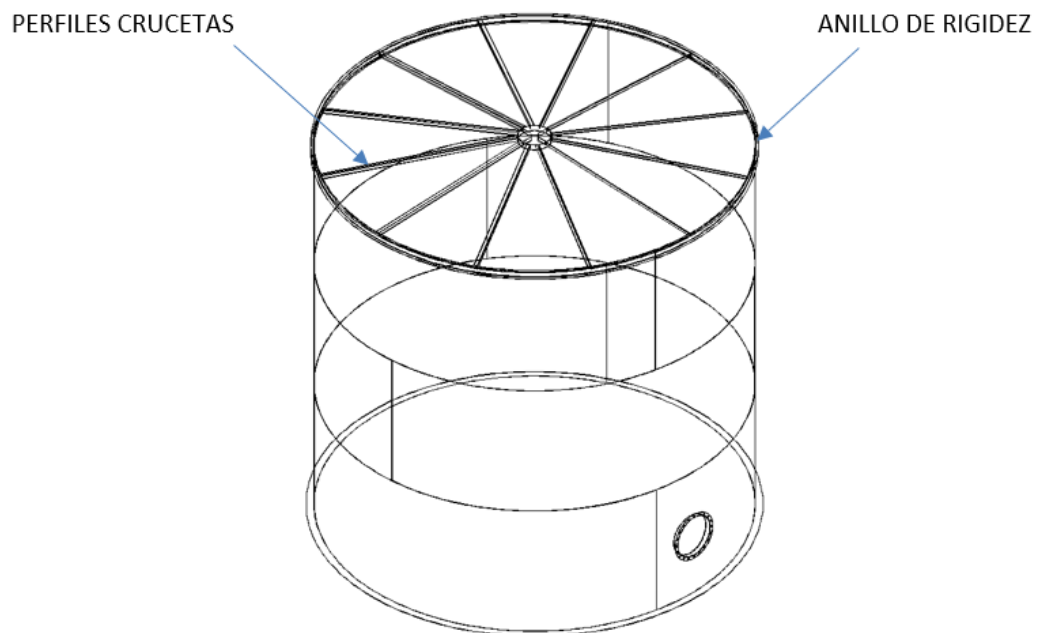
FIG. N°9: Elementos estructurales del tanque de almacenamiento de agua dulce.
